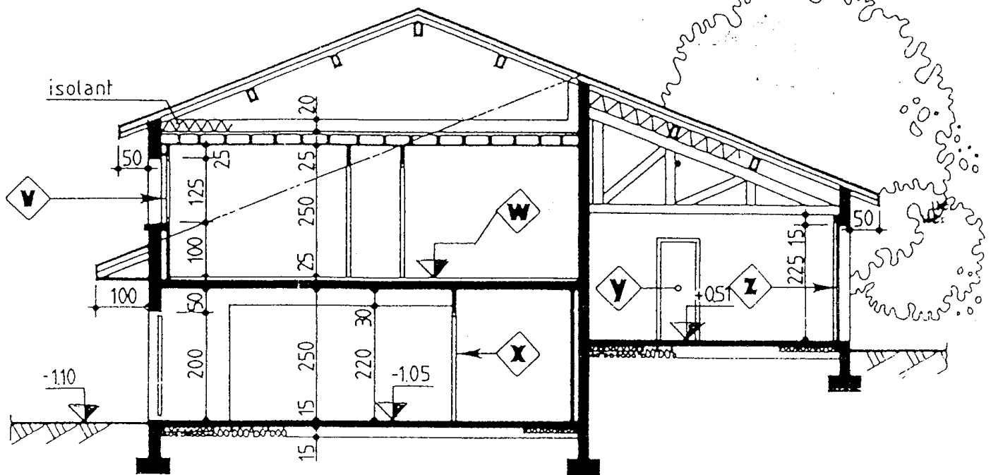
ELEVATION DE LA MAISON EN COUPE A-A
